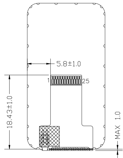
弯折示意图 弯折出货
