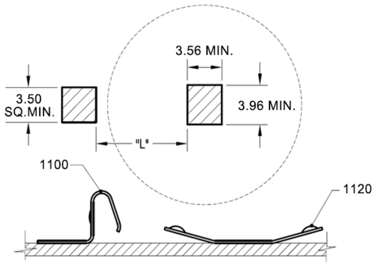
MFG LAYOUT FOR 1100& 1120
