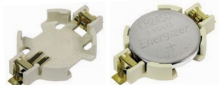
BU2450SM-JJ-G Diameter: 24 mm
