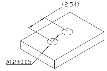
线路板插孔尺寸
