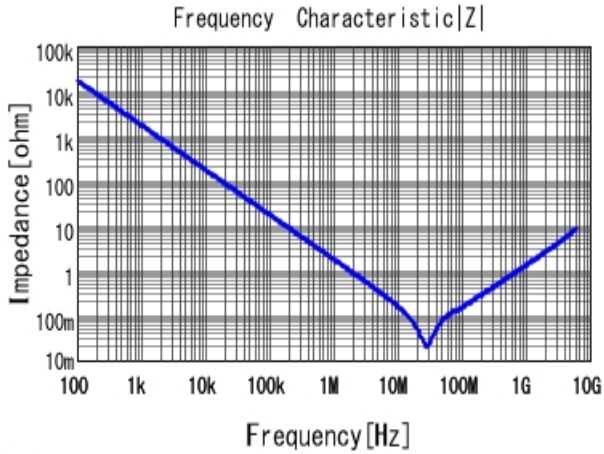
■ GRT155R71H104KE01 |Z| DCOV, 25degC
