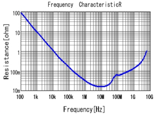
■ GRT155R71H104KE01 R DCOV, 25degC
