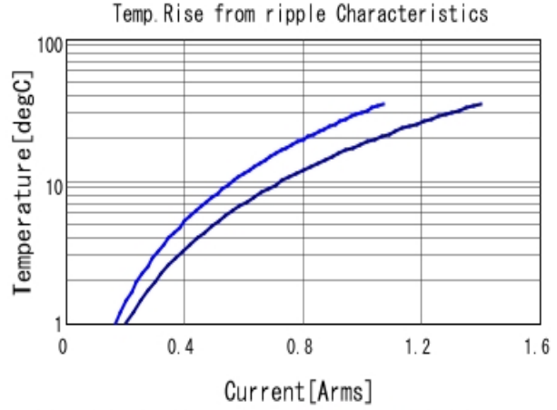
■ GRT155R71H104KE01 Temp. rise ■ 500kHz ■ 1MHz
