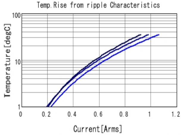
GRM1555C1H120GA01 Temp. rise ■ 500MHz ■ 700MHz ■ 1GHz
