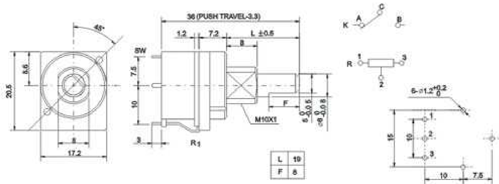
产品尺寸图:
