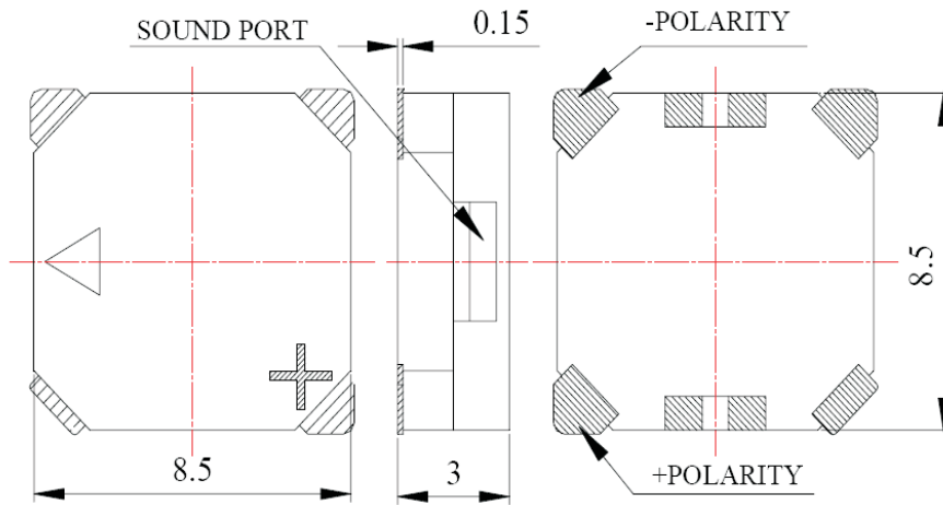
Unit:mm Tol:±0.3
