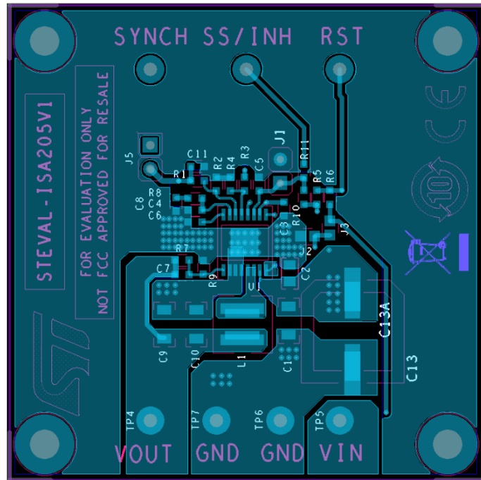
Figure 56. Bottom layer
