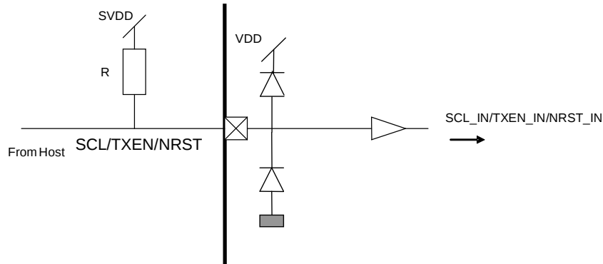
Figure 29: SCL/TXEN/NRST
